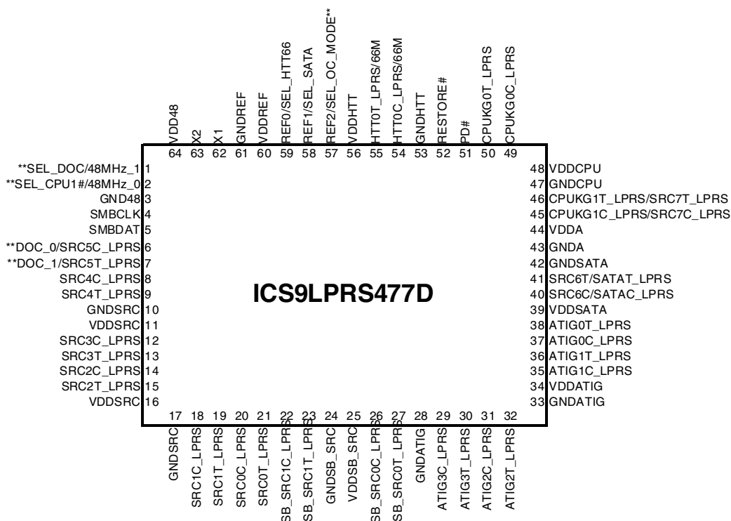
64-Pin MLF
